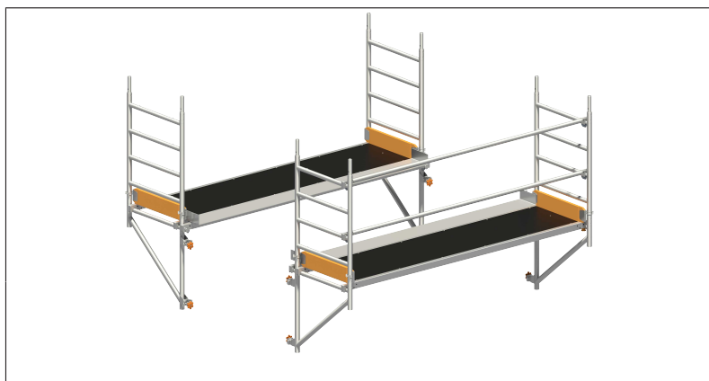
Konsolbelagflächen-Kit Uni Standard und Uni Breit
