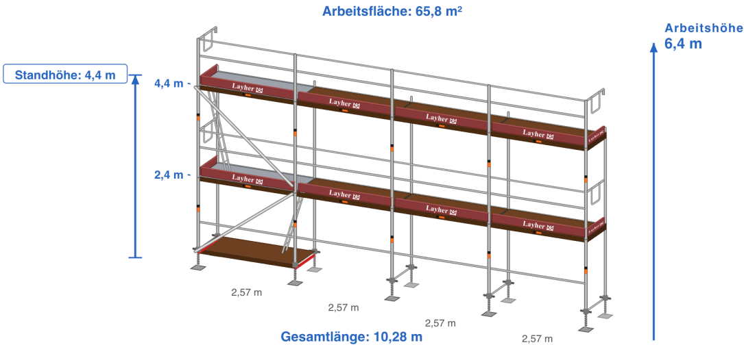
Abbildung: Aufbauschema — verbindlich ist die Materialliste.
