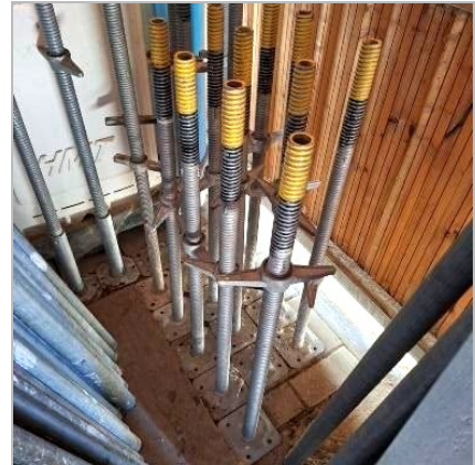
Nr. 248 · Fußspindeln
