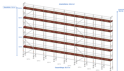
Abbildung: Aufbauschema — verbindlich ist die Materialliste.
