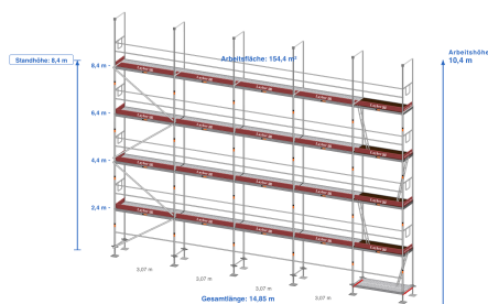
Abbildung: Aufbauschema — verbindlich ist die Materialliste.
