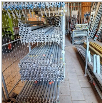
Nr. 146 · AR O-Riegel in Layher Stapelbox (Rohrpalette 125)
