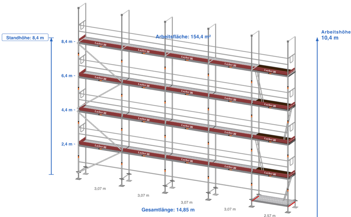
Abbildung: Aufbauschema — verbindlich ist die Materialliste.
