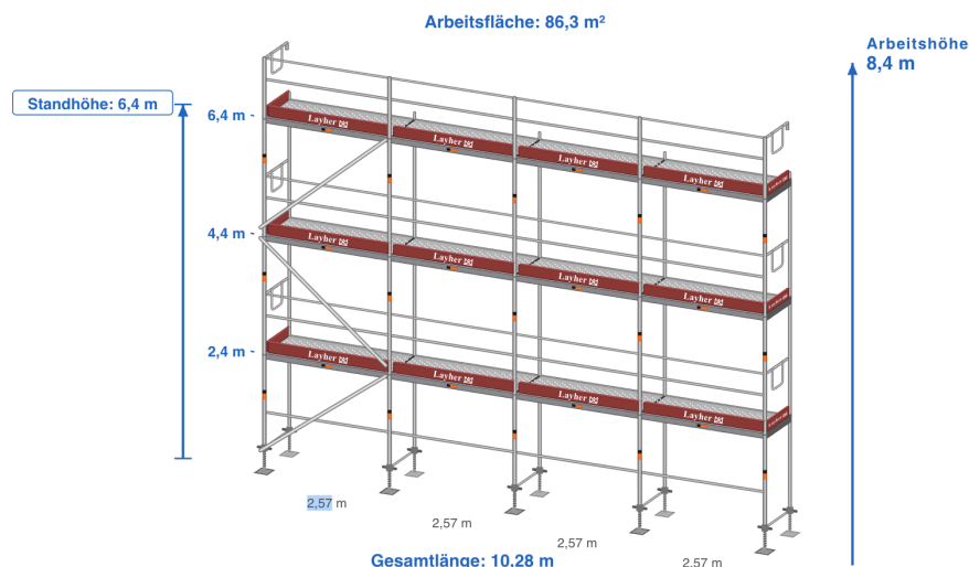
Abbildung: Aufbauschema — verbindlich ist die Materialliste.
