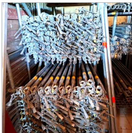
Nr. 217 · Blitz Diagonale
