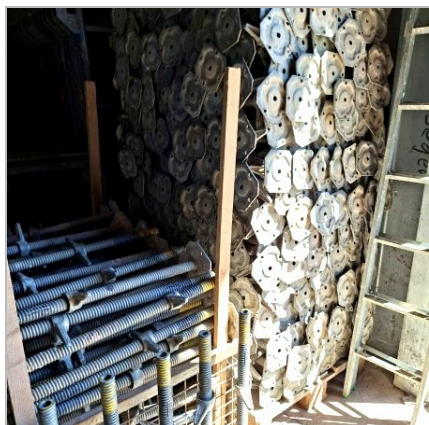
Nr. 175 · Fußspindeln und Fußplatten
