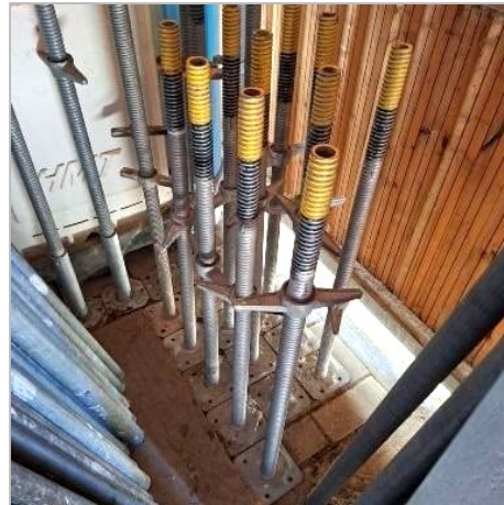
Nr. 248 · Fußspindeln
