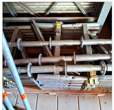
Nr. 158 · AR Anfangsstück lang
