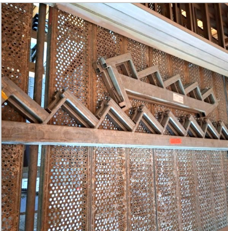
Nr. 256 · U-Treppenwange
